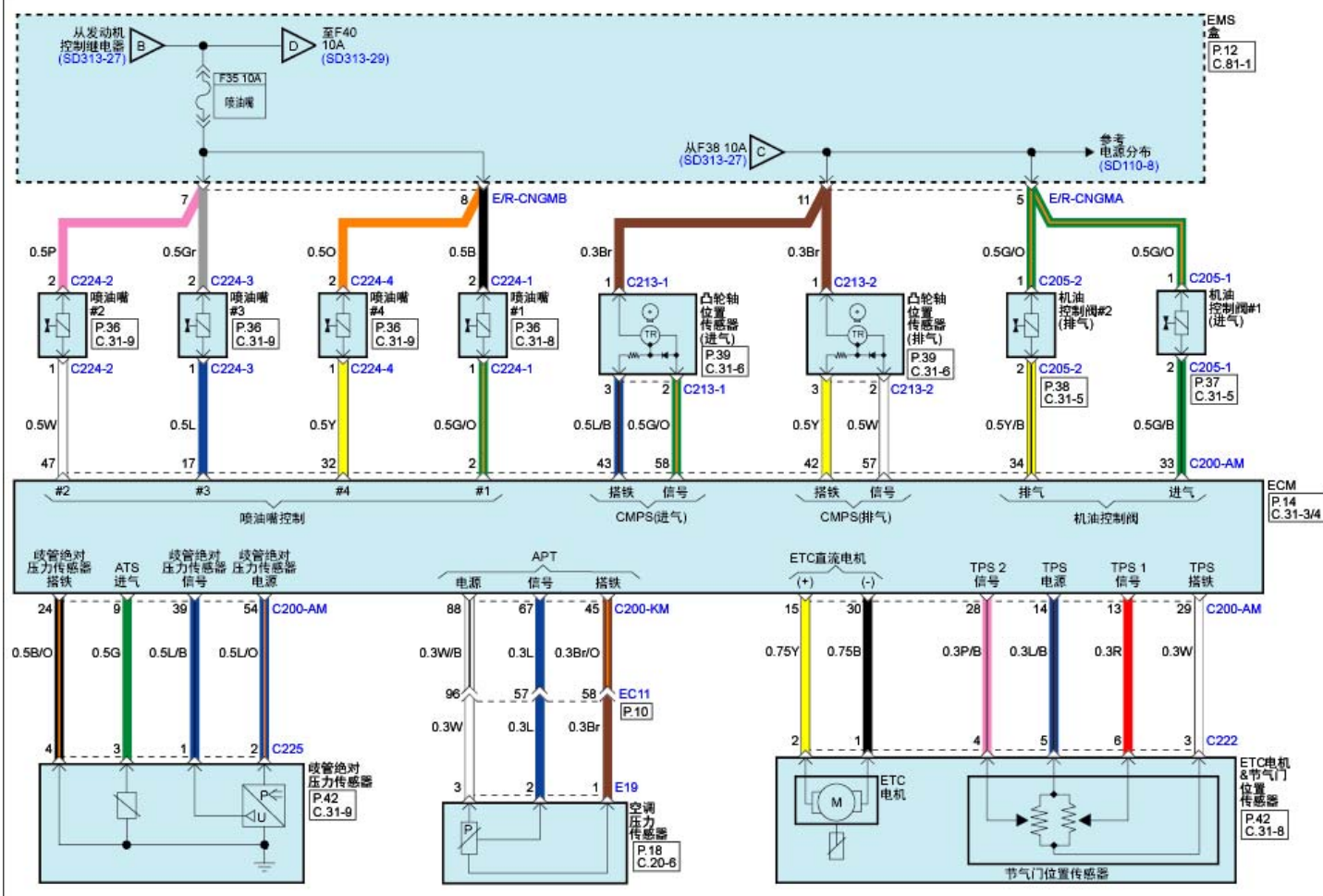
发动机电控系统(G4NA : NU 2.0L MPI M/T)(4)
